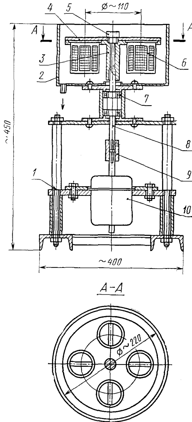
1 — рама; 2 — кожух; 3 — держатель корзинок; 4 — крышка; 5 — прижимной болт; 6 — корзинка; 7 — узел подшипника; 8 — вал; 9 — муфта; 10 — электродвигатель постоянного тока СЛ-369 У/А.
