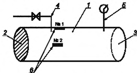
1 — отрезок трубопровода; 2, 3 — герметичные заглушки; 4 — штуцер; 5 — манометр; 6 — зоны измерений (№ 1 и № 2)
