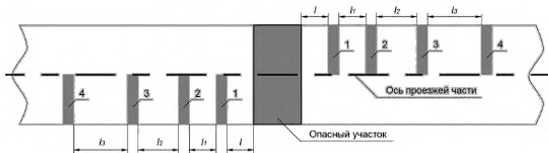
Рисунок А.1 – Пример схемы устройства комплекса ШП, выполненных из цветных покрытий противоскольжения
