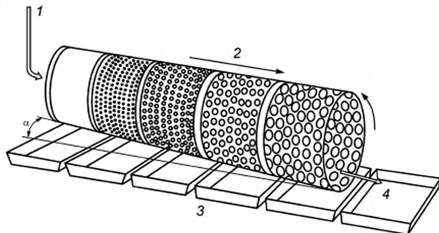
1 — загрузка пробы; 2 — направление увеличения размеров отверстий; 3 — сборные лотки (поддоны); 4 — направление движения пробы
