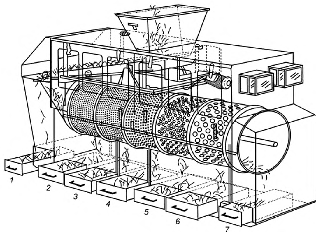
Рисунок А.1 — Пример конструкции ротационного грохота
