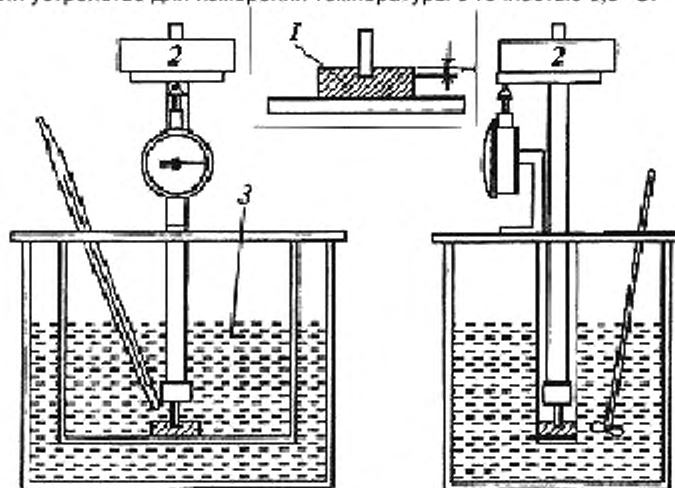
1 – образец; 2 – нагрузка; 3 – масляная ванна Рисунок 2 – Схема прибора
