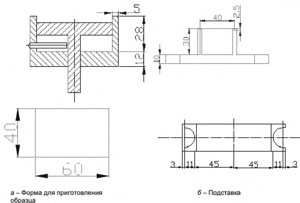
Рисунок 4 – Детали копра
