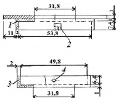
Рисунок 3 – Модернизированный прибор
