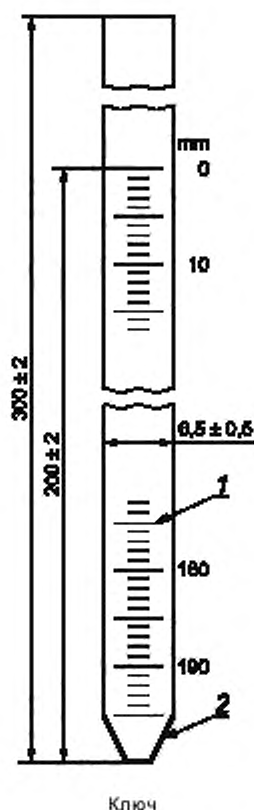
Рисунок 2 — Капиллярная трубка Вестергрена для многократного использования
