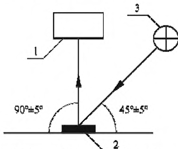
1 – Спектрофотометр или колориметр для измерения координат цветности, спектрофотометр, колориметр или яркомер для измерения коэффициента яркости; 2 – дорожная разметка; 3 – источник света
