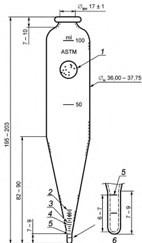
Рисунок 1 — Пробирка ASTM для определения следов осадка
