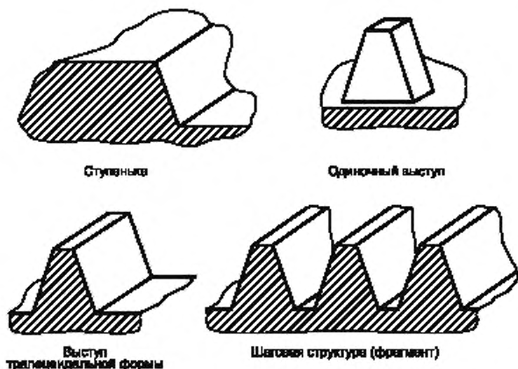
Рисунок 1 — Типовые элементы рельефа рельефной меры
