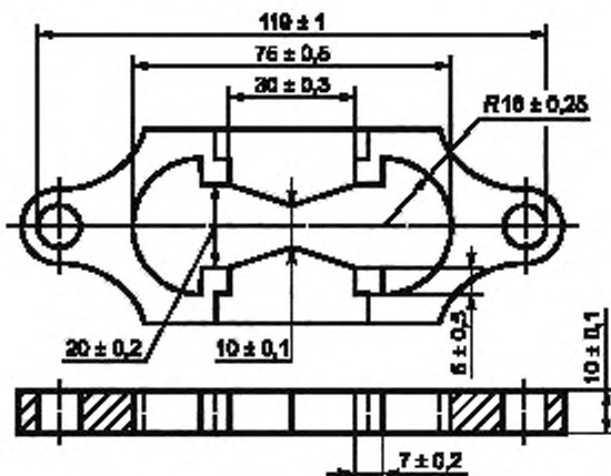
Рисунок 1 — Форма для битума
