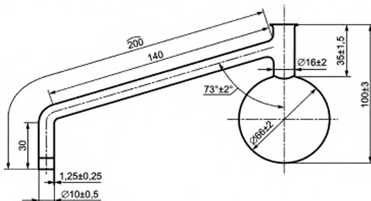
Рисунок 1 — Перегонная колба
