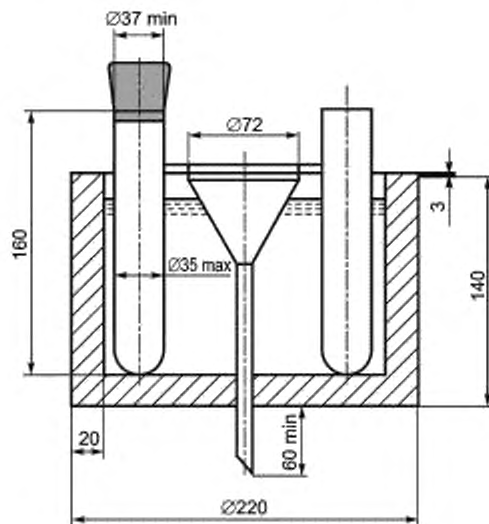
Рисунок 2 — Охлаждающая баня
