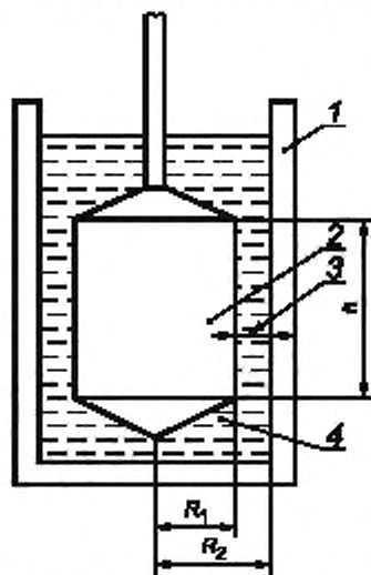
1 — контейнер для битума; 2 — вал; 3 — толщина рабочего слоя битума. 4 — испытуемый битум, R_1 — радиус валика, R_2 — внутренний радиус контейнера
