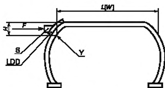
б) Пример изогнутого конструктивного элемента (изогнутой стойки), показывающий приложение нагрузки
