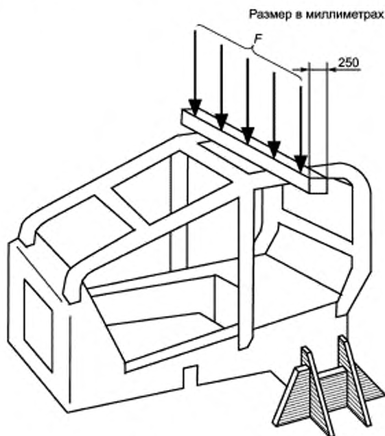
Рисунок 7 — Вертикальное нагружение
