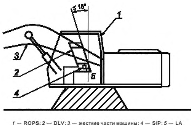
Рисунок 10 — Наклон DLV вперед при продольном нагружении сзади
