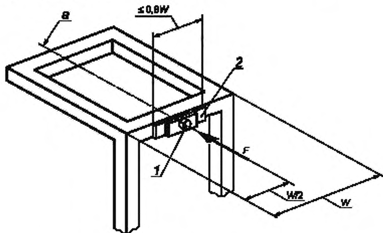
Рисунок 8 — Устройство распределения продольной нагрузки
