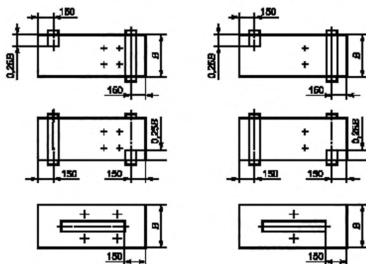
Рисунок Е.1 — Схемы нагружения жесткой балки перекрытия при испытании на изгиб с кручением
