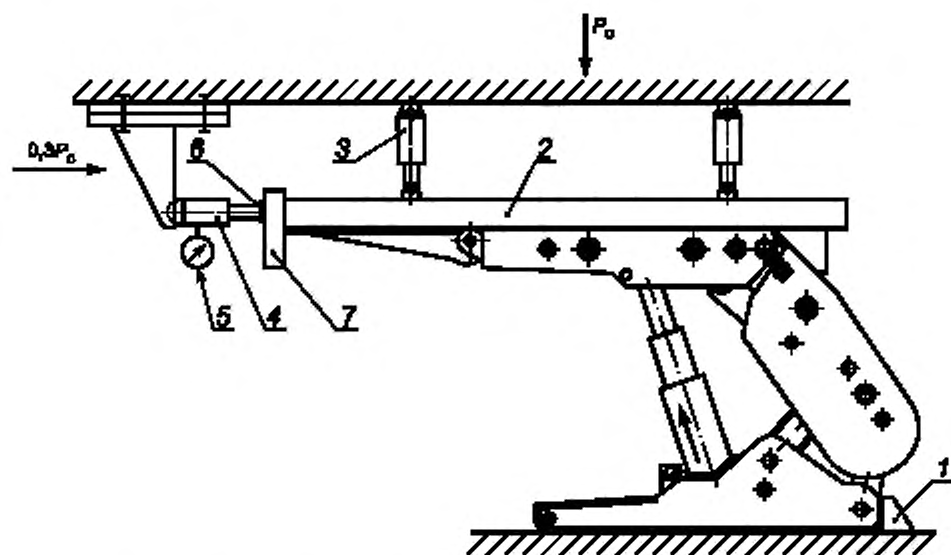
1 — упор; 2 — рама; 3, 4 — гидродомкраты; 5 — манометр; 6 — тензопора; 7 — упор
