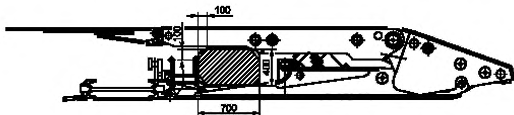
Рисунок 1 — Минимальные размеры прохода (размеры в мм)
