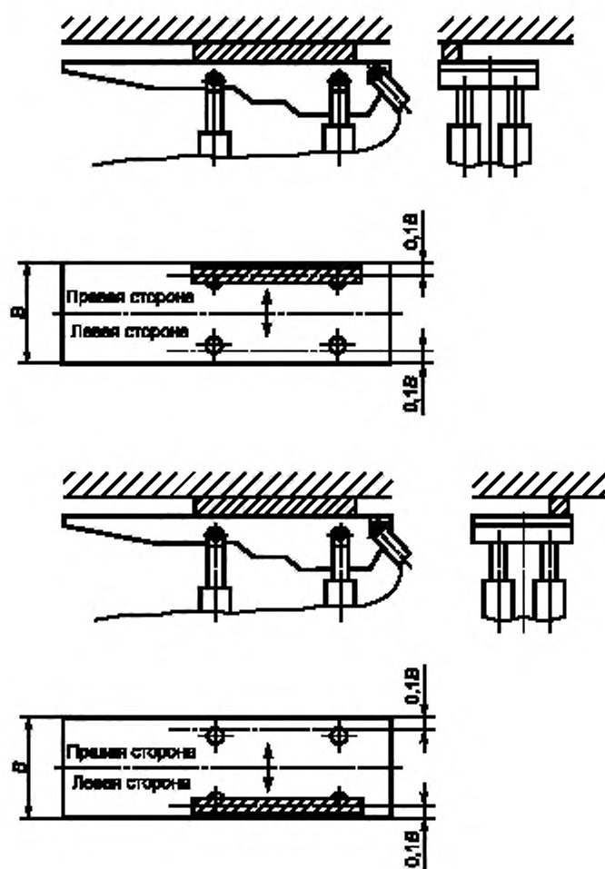
Рисунок Л.1 — Схемы испытаний на внецентренную нагрузку четырёхстоечной секции крепи
