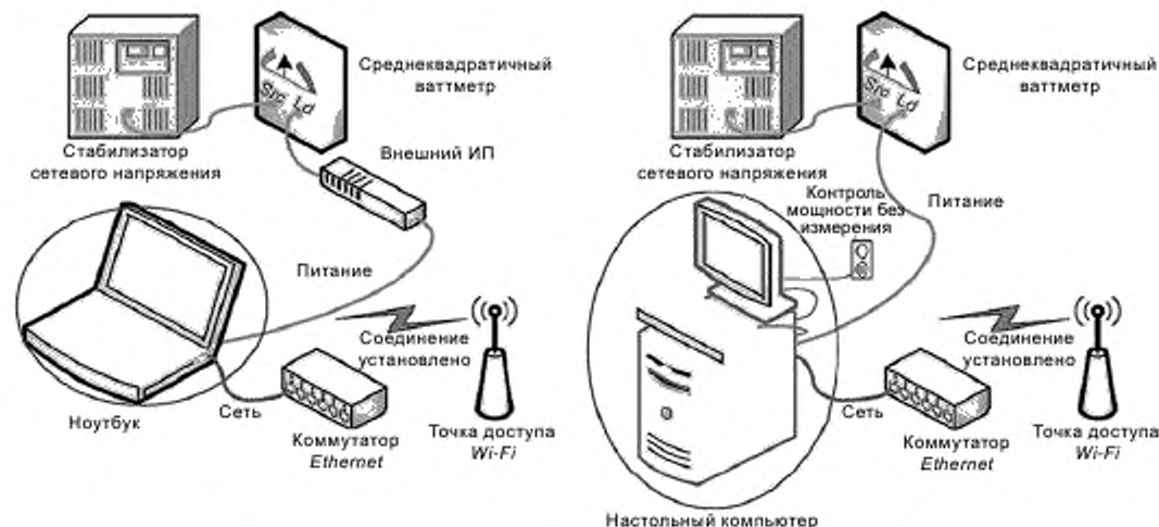
Рисунок 1 — Типичная испытательная установка
