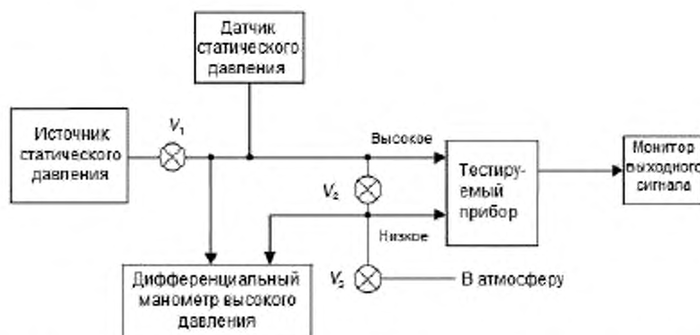
Рисунок 4 – Установка, рекомендованная для проведения тестовых испытаний по определению влияния статического давления
