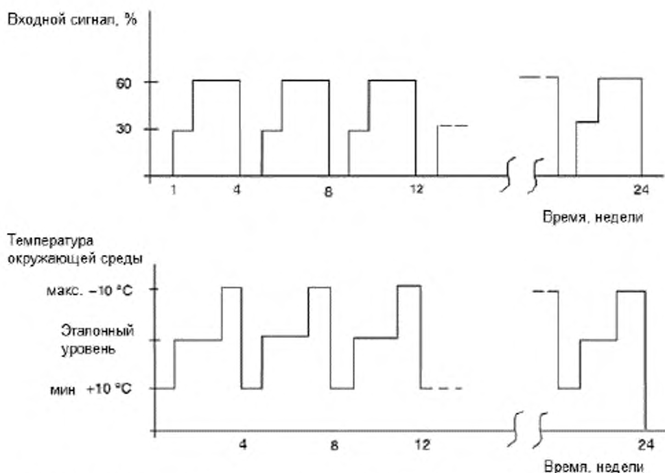
Рисунок 5 – Временные диаграммы изменений входных сигналов и температуры окружающей среды
