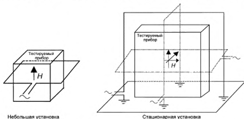
Рисунок 3а – Пример применения тестового магнитного поля с помощью иммерсионного метода
