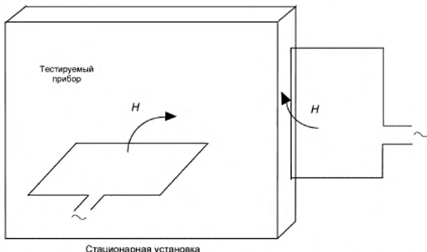
Рисунок 3б – Пример применения тестового магнитного поля с помощью метода приближения
