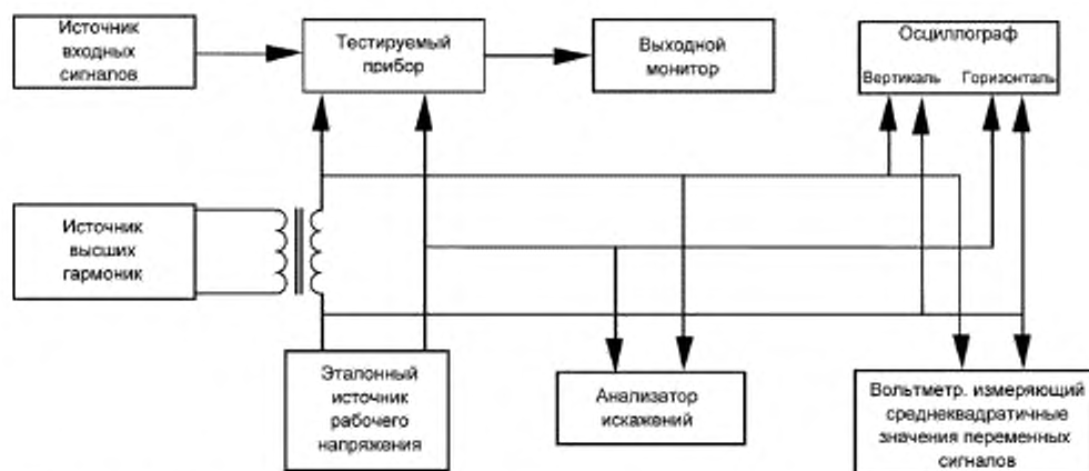
Рисунок 2 – Схема установки для проведения тестовых испытаний для определения влияния гармонических искажений сигнала источника электропитания переменного тока
