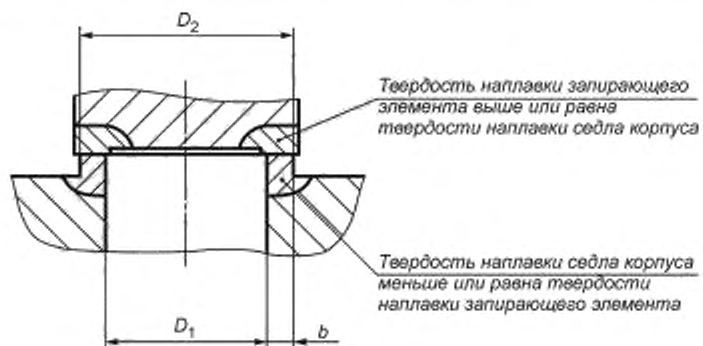
Рисунок Е.1 — Плоское уплотнение в затворе
