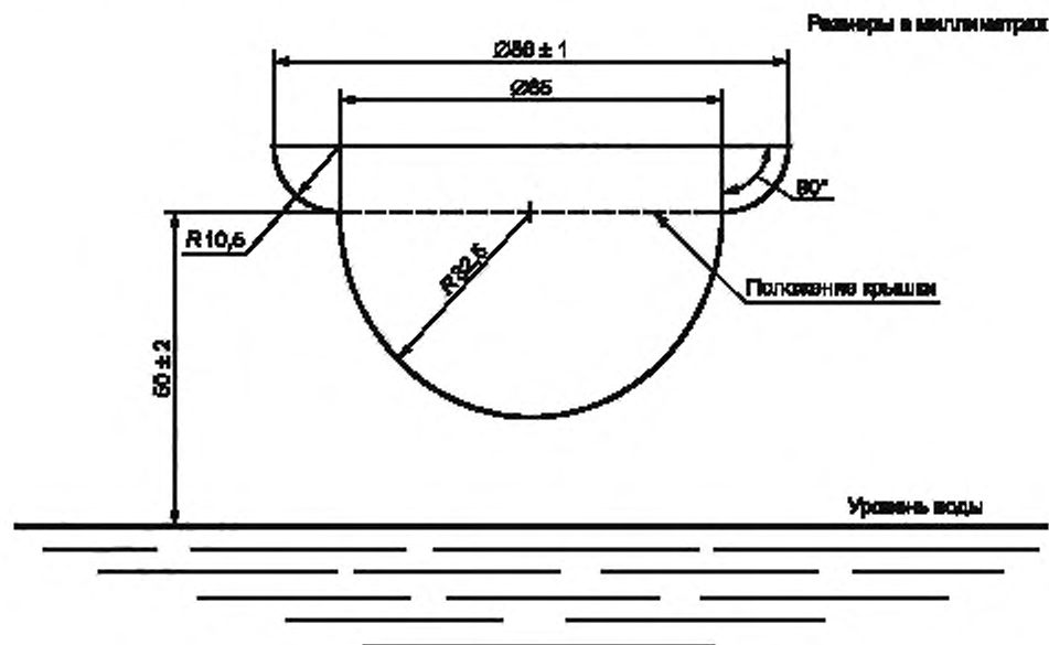
Рисунок — Чашка для выпаривания на водяной бане
