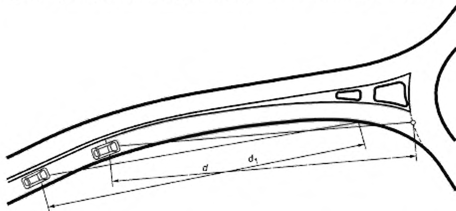
Рисунок Б.1 — Схема для измерения расстояния видимости при въезде на кольцевое пересечение
