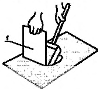
г - режущая пластина, д - детальное изображение отбора точечной пробы в одной из 20 частей с использованием режущей пластины, показанной на рисунке
