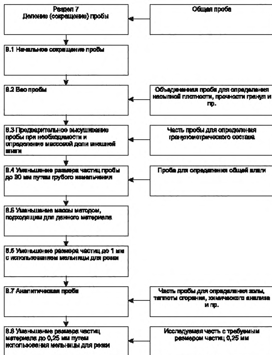
Рисунок 5 – Схема сокращения пробы
