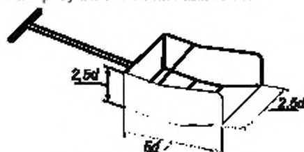
Рисунок 3 – Пример лопаты
