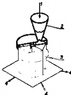
1 - подающий механизм; 2 - воронка; 3 - вращающийся приемник; 4 - разделитель проб
