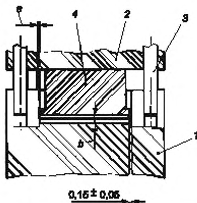
1 – основание; 2 – верхняя рама; 3 – направляющие; 4 – поршень; а – уклон по всему периметру 1°; b – режущие края по всему периметру
