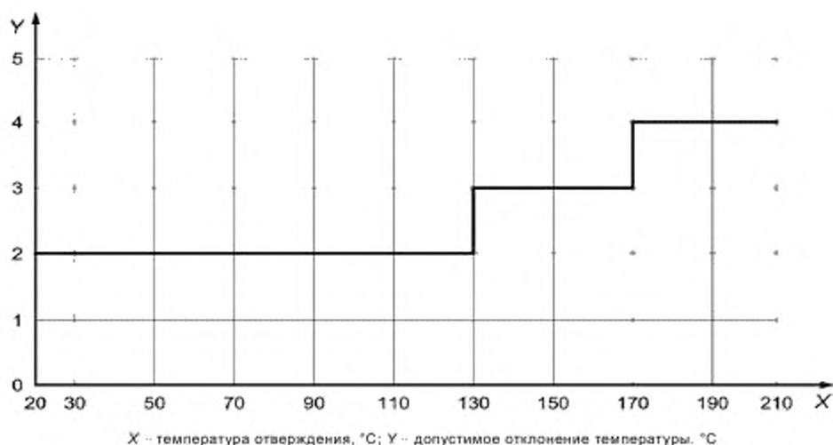
X – температура отверждения, °C; Y – допустимое отклонение температуры, °C Рисунок 5 – Примеры допустимых отклонений температуры от температуры отверждения
