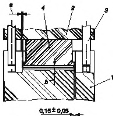
Рисунок 1 – Пресс для формования
