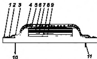
Рисунок 3 – Схема формования пластин в автоклаве
