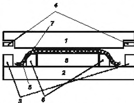
1 – верхняя пластина; 2 – опорная пластина; 3 – направляющие вставки; 4 – вставки заданной толщины; 5 – влитывающий материал; 6 – металлические брусья; 7 – мембранное полотно; 8 – уложенные слои препрега
