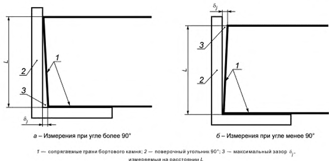
Рисунок 1 — Схема контроля взаимной перпендикулярности граней бортового камня
