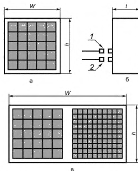
а, в — виды спереди, б — вид сбоку; t — ввод питания; 2 — ввод управления; w — ширина; h — высота; t — толщина. Закрашенные прямоугольники являются эквивалентными областями элементов и образуют область проверки светотехнических характеристик.
