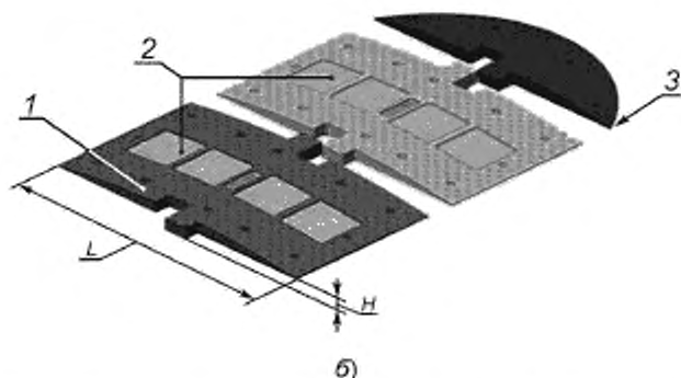
а — общий вид ИНС, состоящих из основных и краевых элементов; б — общий вид фрагментов ИНС, состоящих из основных и краевых элементов: 1 — основной элемент; 2 — световозвращающие элементы; 3 — краевой элемент, L — длина хорды, H — высота гребня
