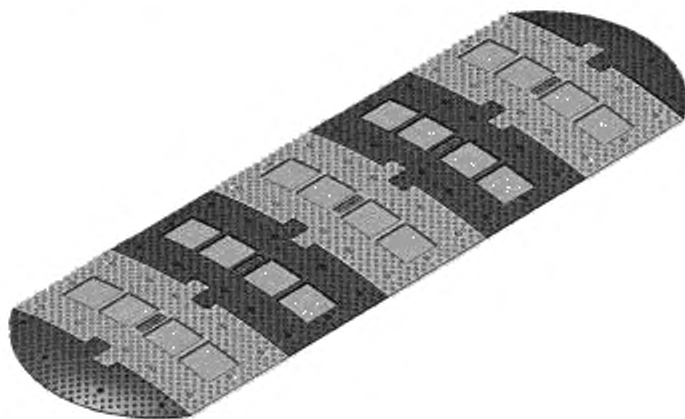
Рисунок 1 — Типовая ИНС
