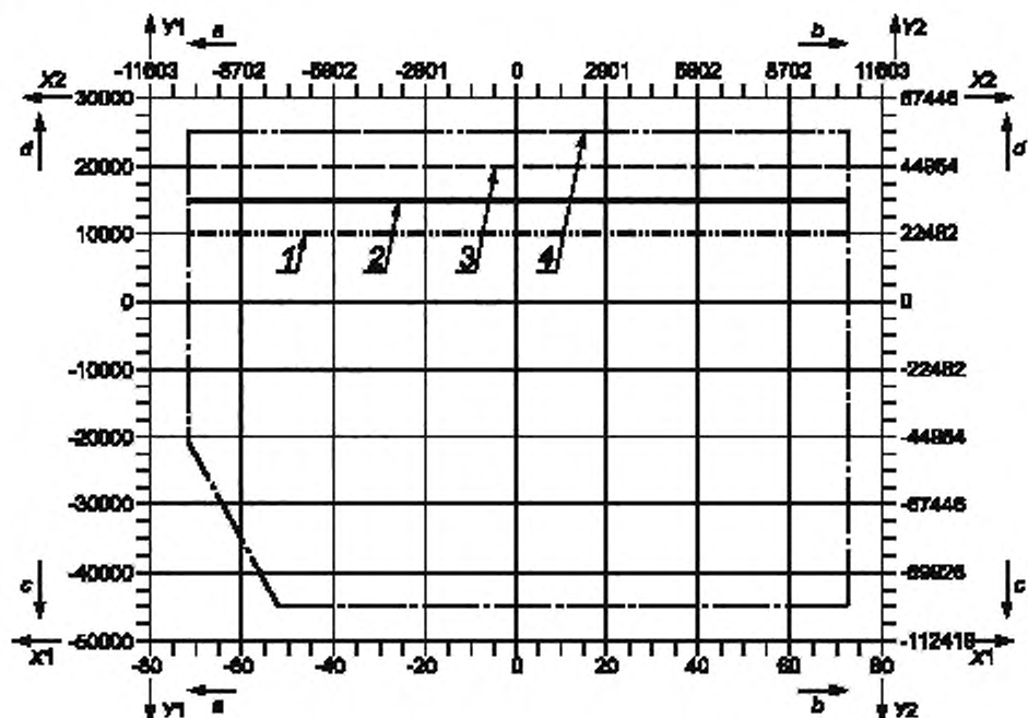
X1 — давление, МПа, X2 — давление, фунт/дюйм 2 , Y1 — сила, даН; Y2 — сила, фунт; 1 — область для 10 000 даН (212 462 фунт) срез. кольцо; 2 — область для 15 000 даН (33 723 фунт) срез. кольцо; 3 — область для 20 000 даН (44 964 фунт) срез. кольцо; 4 — область для 25 000 даН (956 205 фунт) срез. кольца; а — выше, b — ниже; c — сжатие; d — растяжение
