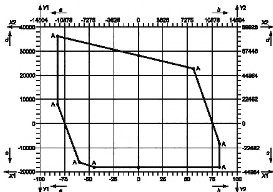
Рисунок 1 — Пример номинальных значений рабочих характеристик
