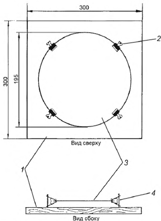
Рисунок 1 — Держатель бумаги для испытания
