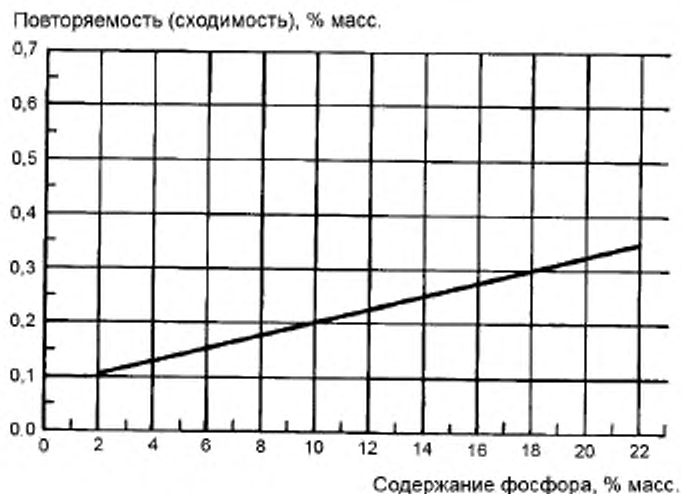
Рисунок 2 – Повторяемость (сходимость) результатов испытаний, полученных гравиметрическим методом
