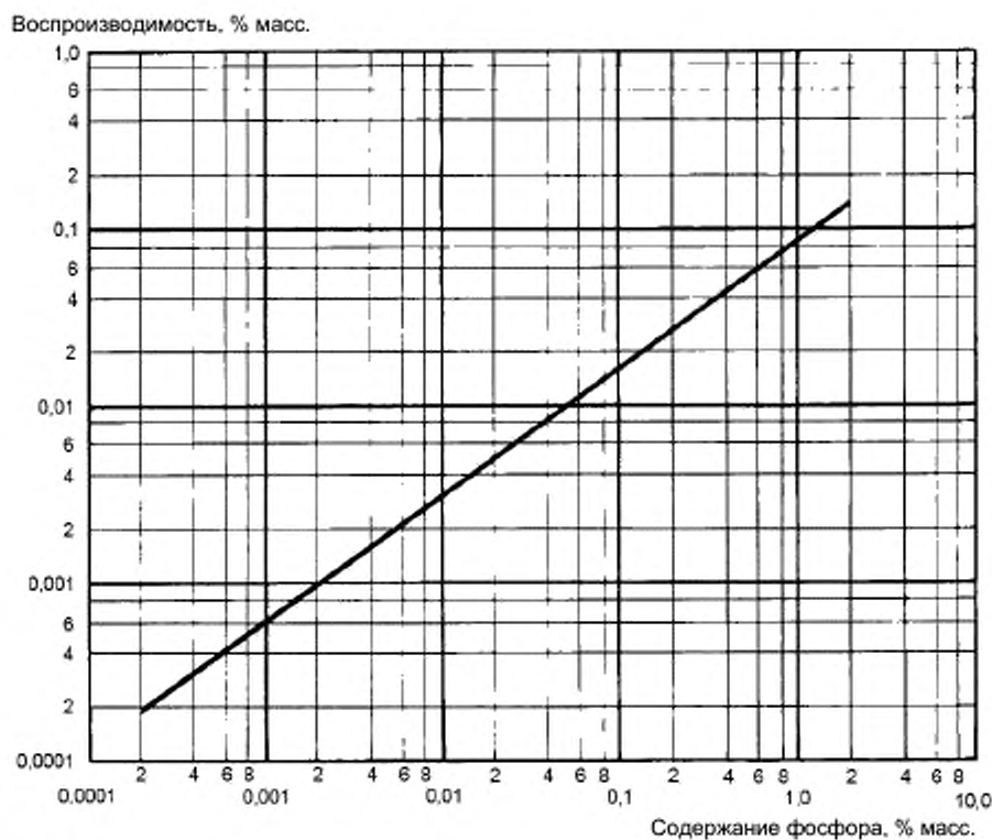
Рисунок 3 – Воспроизводимость результатов испытаний, полученных фотометрическим методом
