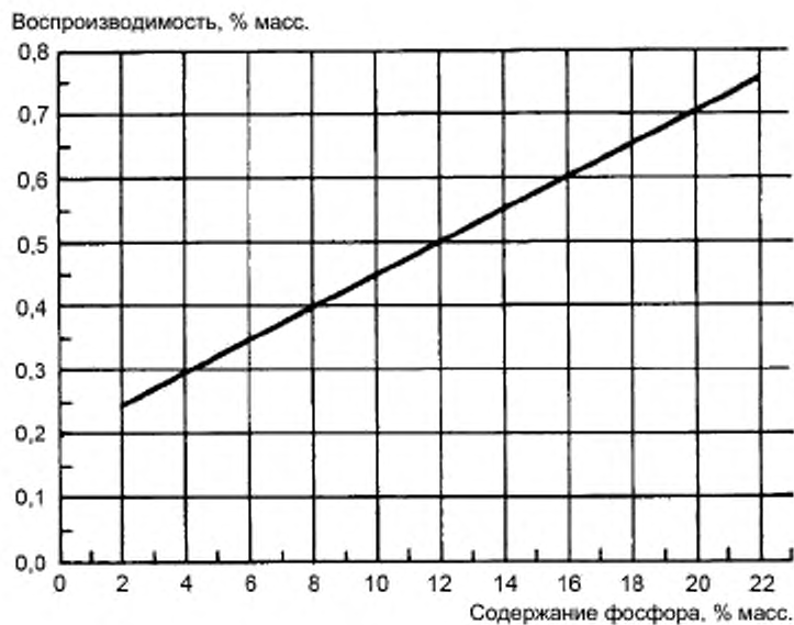
Рисунок 4 – Воспроизводимость результатов испытаний, полученных гравиметрическим методом
