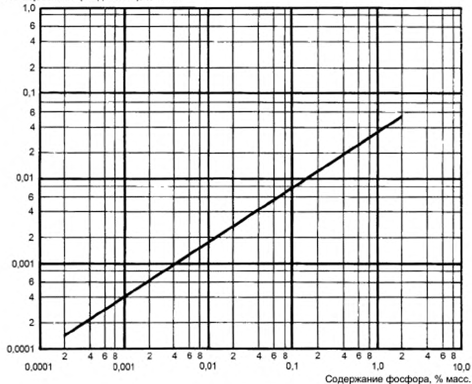
Рисунок 1 – Повторяемость (сходимость) результатов испытаний, полученных фотометрическим методом
