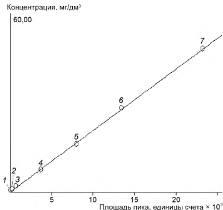
Рисунок 3 – Типичный калибровочный график сульфата
