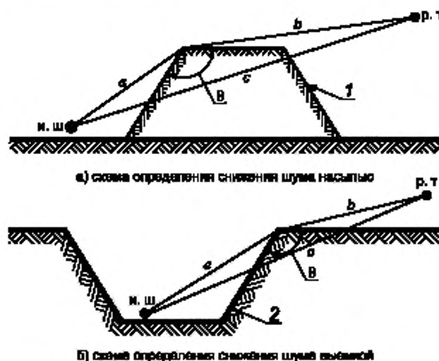
Рисунок 5 — Схема определения снижения шума
