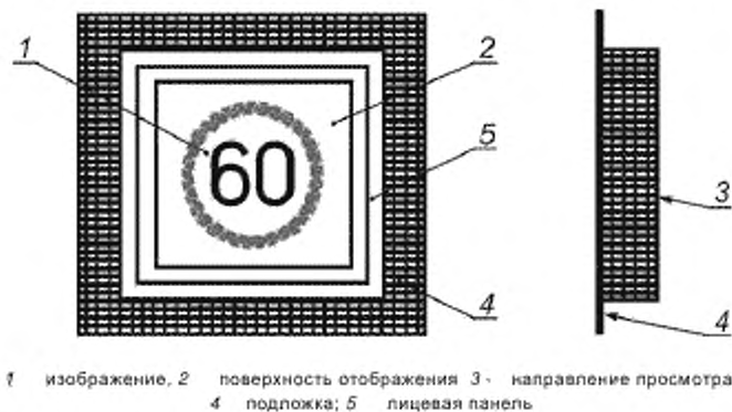
Рисунок А.1 — Основные элементы светотехнического дорожного знака переменной информации
