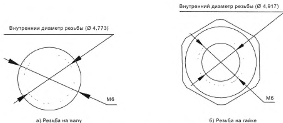
Рисунок 2 — Примеры ЭМД с резьбой М6 согласно ГОСТ 24705
