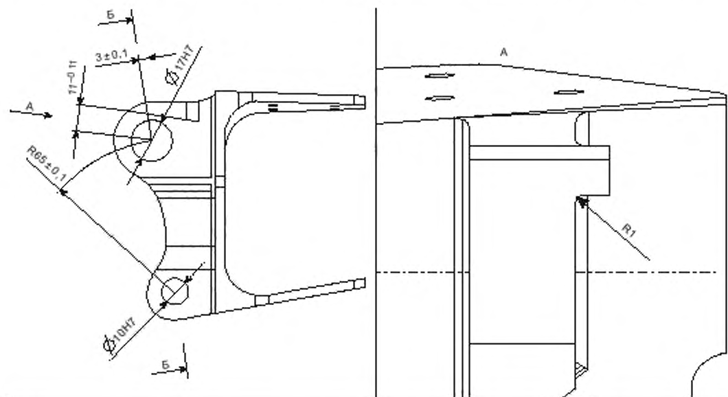
Рисунок В.1 — Пример выполнения дополнительного вида
