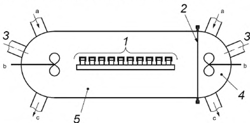
1 – 10 ЛОС/веществ; 2 – перегородка из материала емкости; 3 – область отбора проб; 4 – вторая часть камеры; 5 – первая часть камеры; а – подача чистого воздуха; б – устройство для перемешивания; с – выпуск отработанного воздуха.
