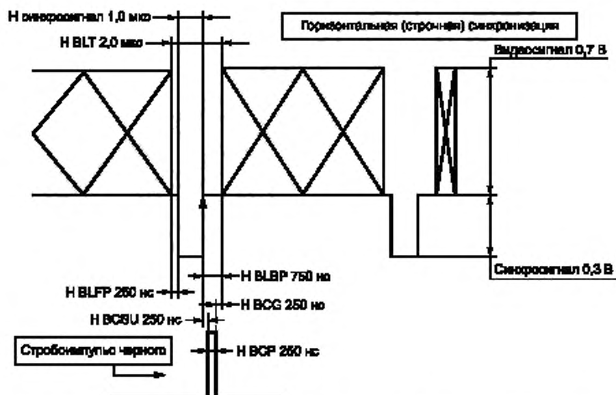
а — Соотношение стробирующего импульса черного к импульсу горизонтального синхросигнала при минимальном значении 500 нс «задней площадки гасящего импульса»
