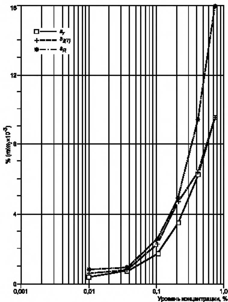
Рисунок D.3 — Содержание ванадия в стали. Стандартные отклонения повторяемости s_r , промежуточной прецизионности с изменяющимся фактором времени s_{R(1)} и воспроизводимости s_R как функции уровня концентрации
