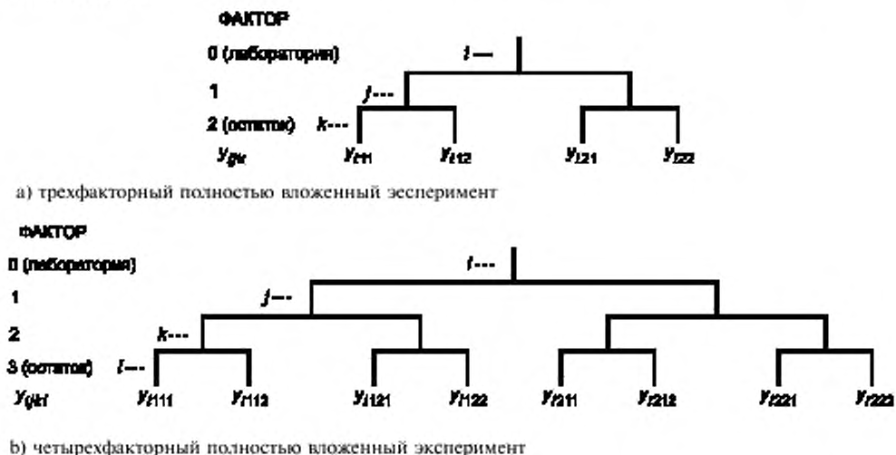
Рисунок 1 — Схемы трех- и четырехфакторных полностью вложенных экспериментов
