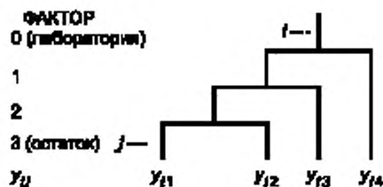
Рисунок 2 — Схема четырехфакторного ступенчато вложенного эксперимента
