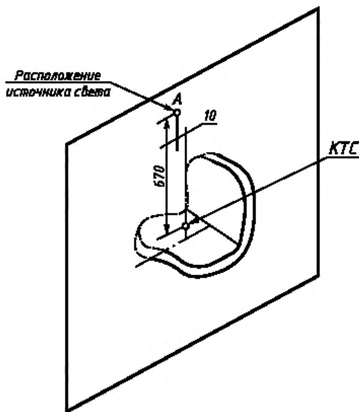
Рисунок 2 — Расположение координат источника света и глаз оператора
