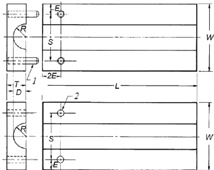
1 – штифт; 2 – отверстие; T – толщина пластины адаптера для захватов; D – радиус паза; R – радиус образца; E – расстояние от края адаптера для захватов до центра отверстия для штифта; S – расстояние между центрами отверстий для штифтов; L – длина адаптера для захватов; W – ширина адаптера для захватов
