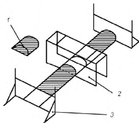
1 — разовая проба, 2 — рамка для отбора проб; 3 — конечные пластины
