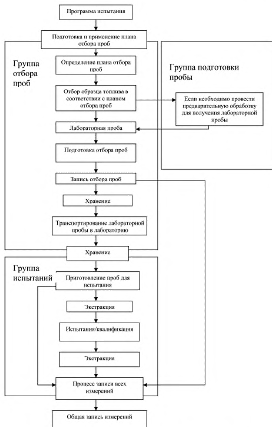
Рисунок 1 — Связи между существенными элементами программы испытания
