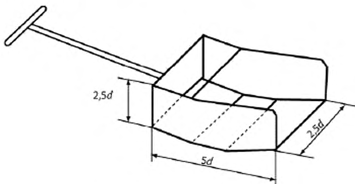
Рисунок 4 — Образец лопаты
