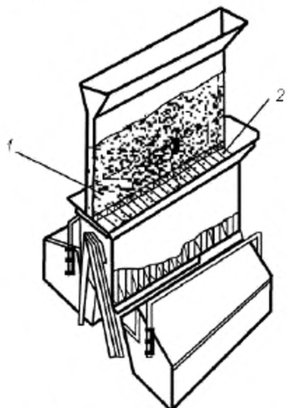
1 — проба; 2 — прорезь размером по крайней мере в 3 раза большим максимального размера материала
