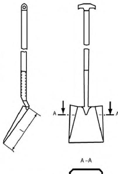
Рисунок 4 — Образец лопаты
