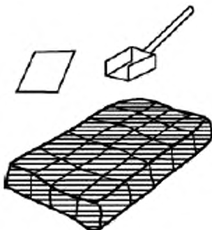
в) Зачерпывание случайных проб из каждой из 20 частей, совок вставляют до дна слоя пробы. Объединяют 20 зачерпков в отдельную пробу
