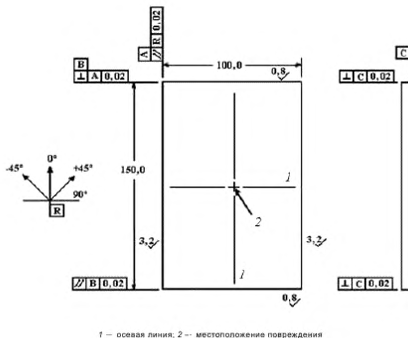
Рисунок 5 — Образец для испытаний ПК на удар
