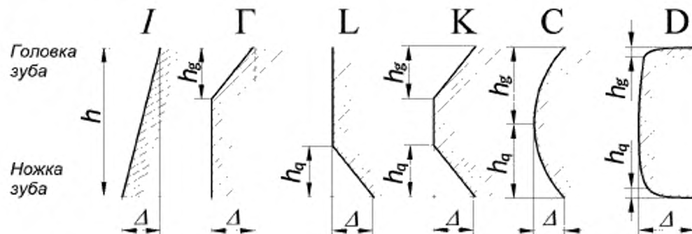
Рисунок ДА.3 — Типы диаграмм модификации профиля в виде отклонения от эвольвенты
