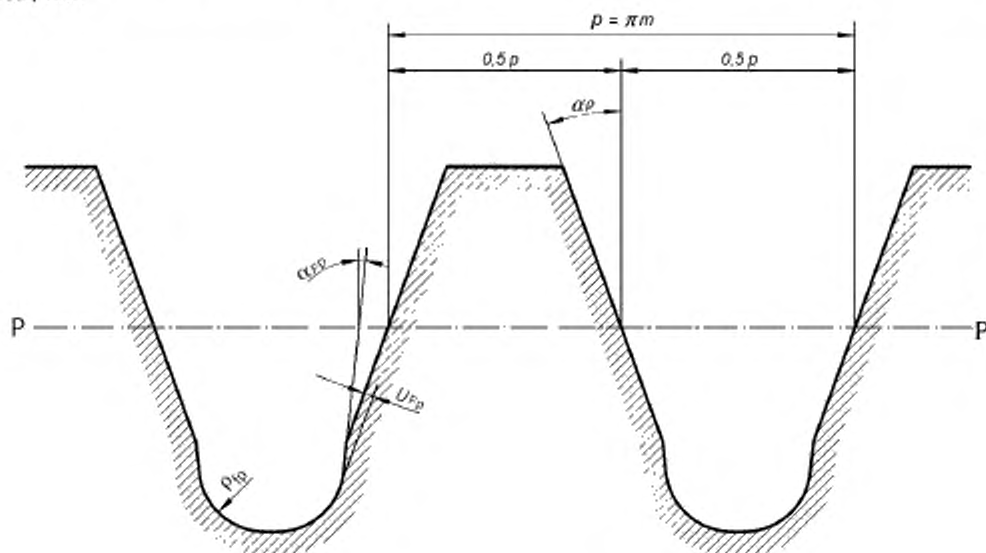
Рисунок А.1 — Исходный контур с поднутрением
