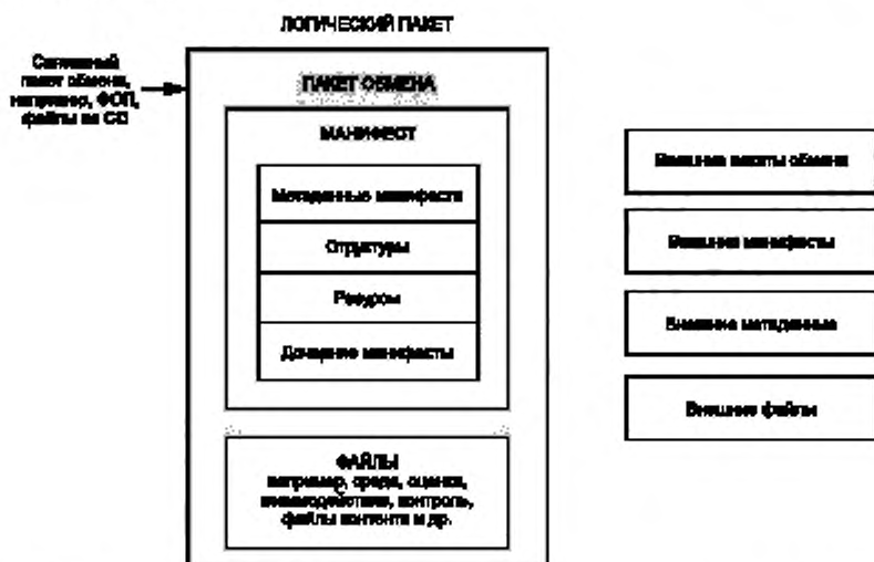
Рисунок 1 — Схематическое представление концептуальной модели упаковки контента (CPCM)
