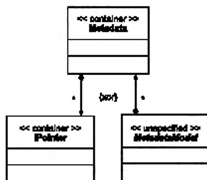
Рисунок 6 — Упрощенное представление класса Metadata PIM
