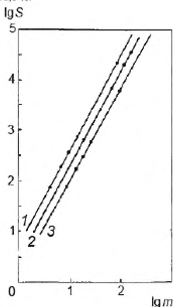
\lg S — десятичный логарифм площади пика ССС; \lg m — десятичный логарифм массы ССС; 1 — сероводород; 2 — метилмеркаптан; 3 — этилмеркаптан
