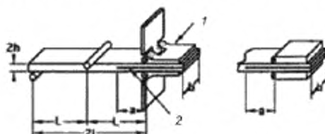
1 – шарнир; 2 – расслаивание
