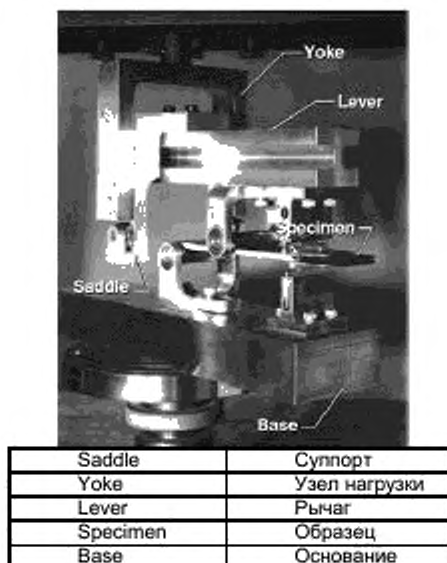
Рисунок 5 – Оснастка для по смешанной моде
