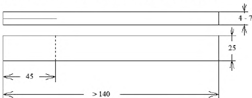
Рисунок 2 – Эскиз образца в форме двухконсольной балки
