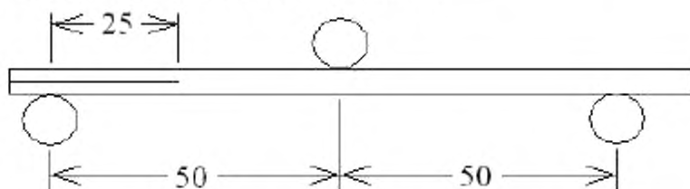
Рисунок 5 – Начальное положение образца на испытательной оснастке
