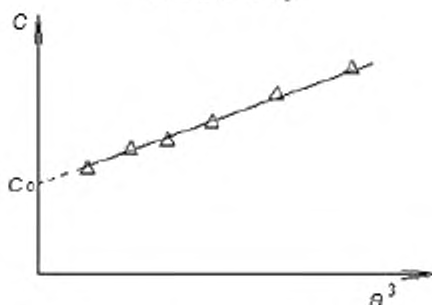
Рисунок 4 – Зависимость податливости образца от длины трещины
