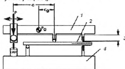
1 – рычаг; 2 – образец испытаний; 3 – нагрузочная высота; 4 – основание Рисунок 1 – Оснастка для испытаний по смешанной моде нагружения I + II
