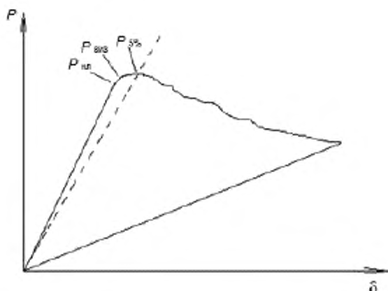
Рисунок 1 – Типовая диаграмма нагрузка – перемещение
