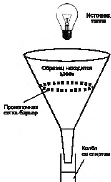
Рисунок Г.1 – Устройство для выделения типа Туллгрена
