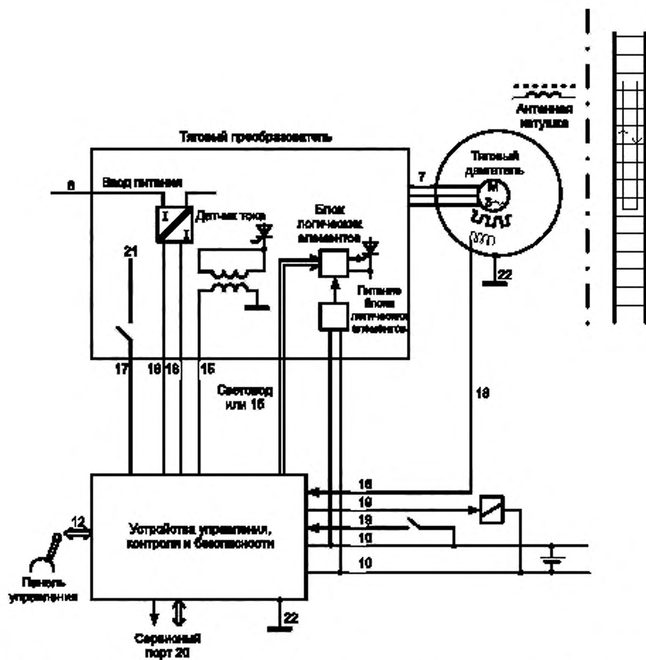
Рисунок А.8 — Дополнительные порты тягового преобразователя тока и электронных схем управления
