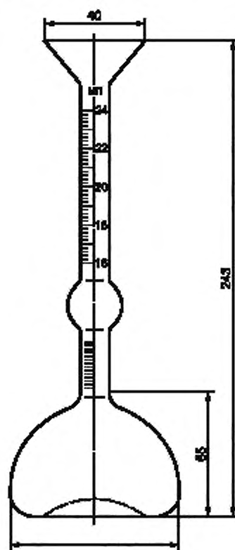
Рисунок 1 — Прибор Ле-Шателье
