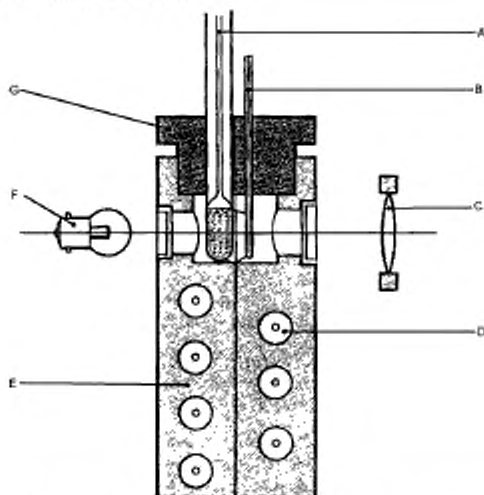
Рисунок 3 — Прибор для определения температуры плавления
