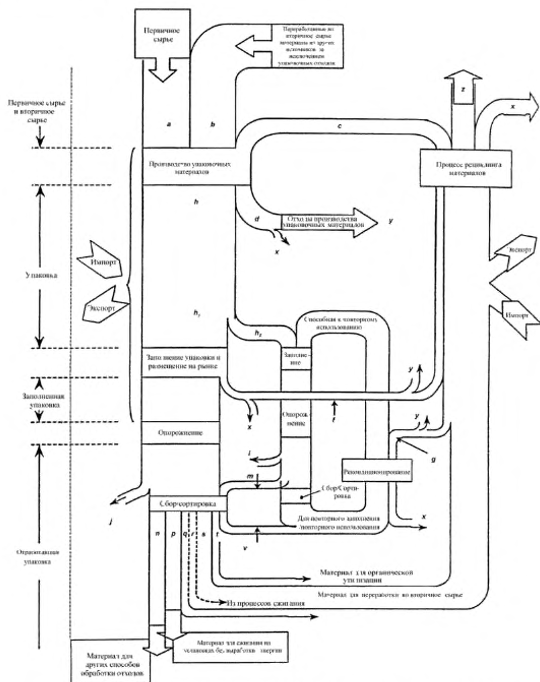
Рисунок А.1 – Поток для переработки упаковки в качестве вторичных материальных ресурсов
