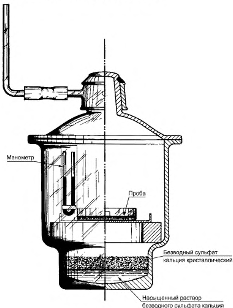
Рисунок 1 — Вакуумный эксикатор
