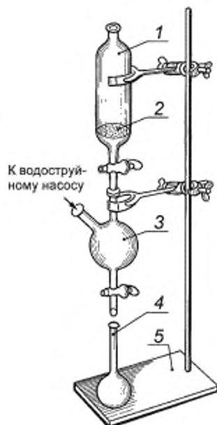
1 — фильтрующая делительная воронка; 2 — аляянный стеклянный фильтр класса ПОР 100 или ПОР 160; 3 — приемник; 4 — мерная колба; 5 — штатив
