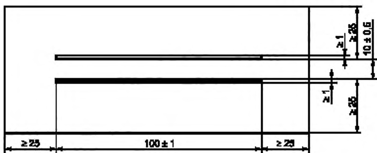
Рисунок G.1 — Испытуемый образец с установленными электродами
